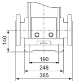
DIN FLANGE(LVR)/F
