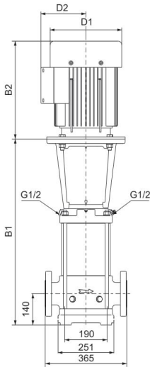
DIN FLANGE(LVS)/F
